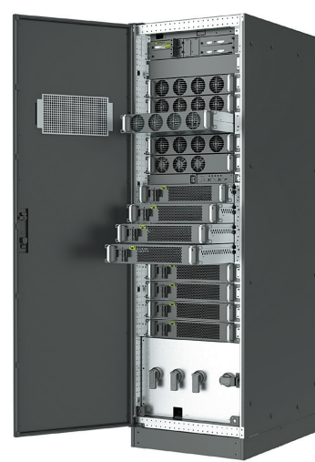
Рис. 2. Масштабування APM2 модулями по 30 кВА
